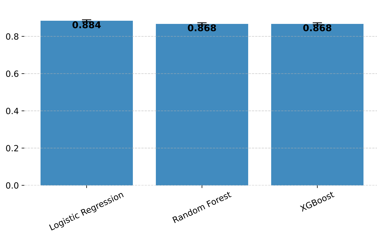
Precision
